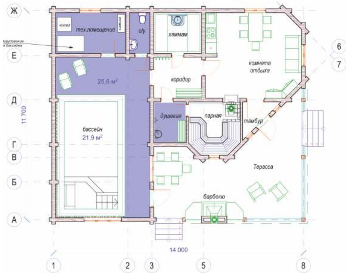
План этажа на отметке ±0,000
